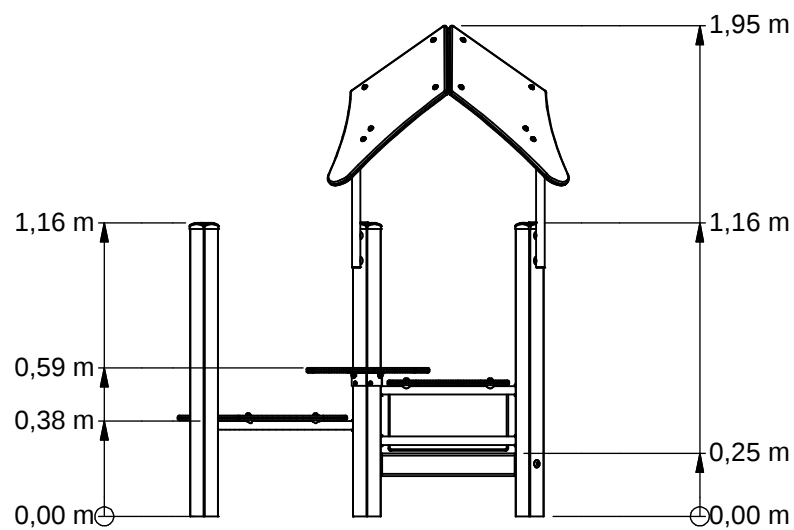
Rechts (Right)
