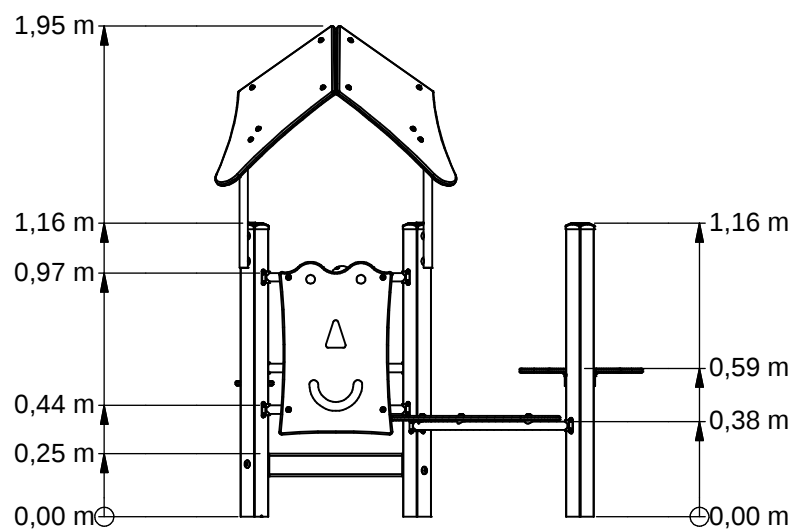
Voor (Front)
