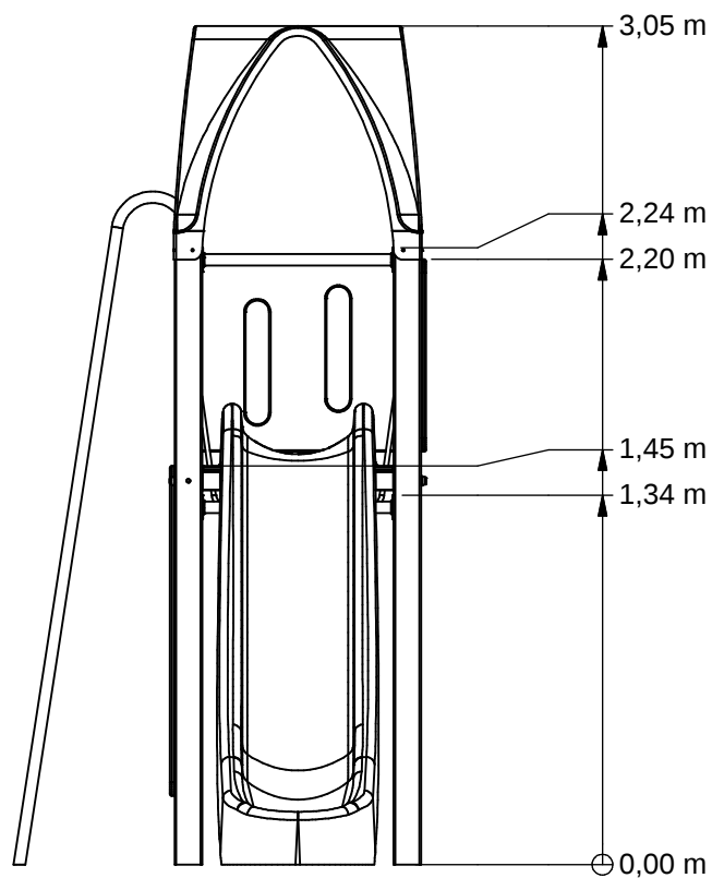
Voor (Front)
