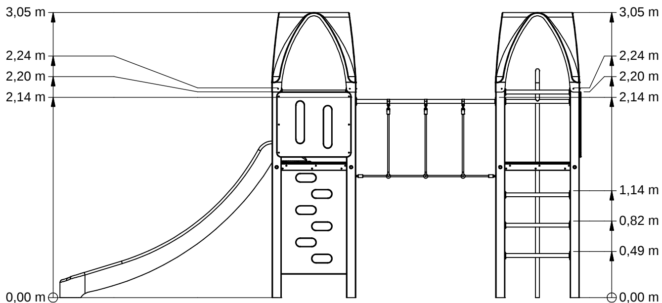
Rechts (Right)
