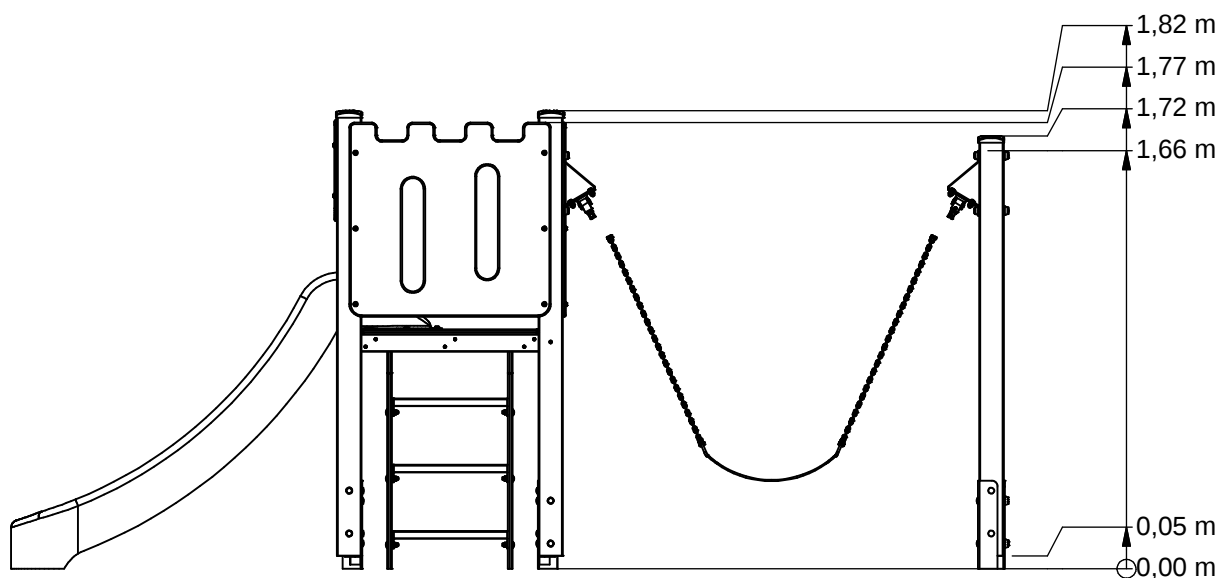
Rechts (Right)
