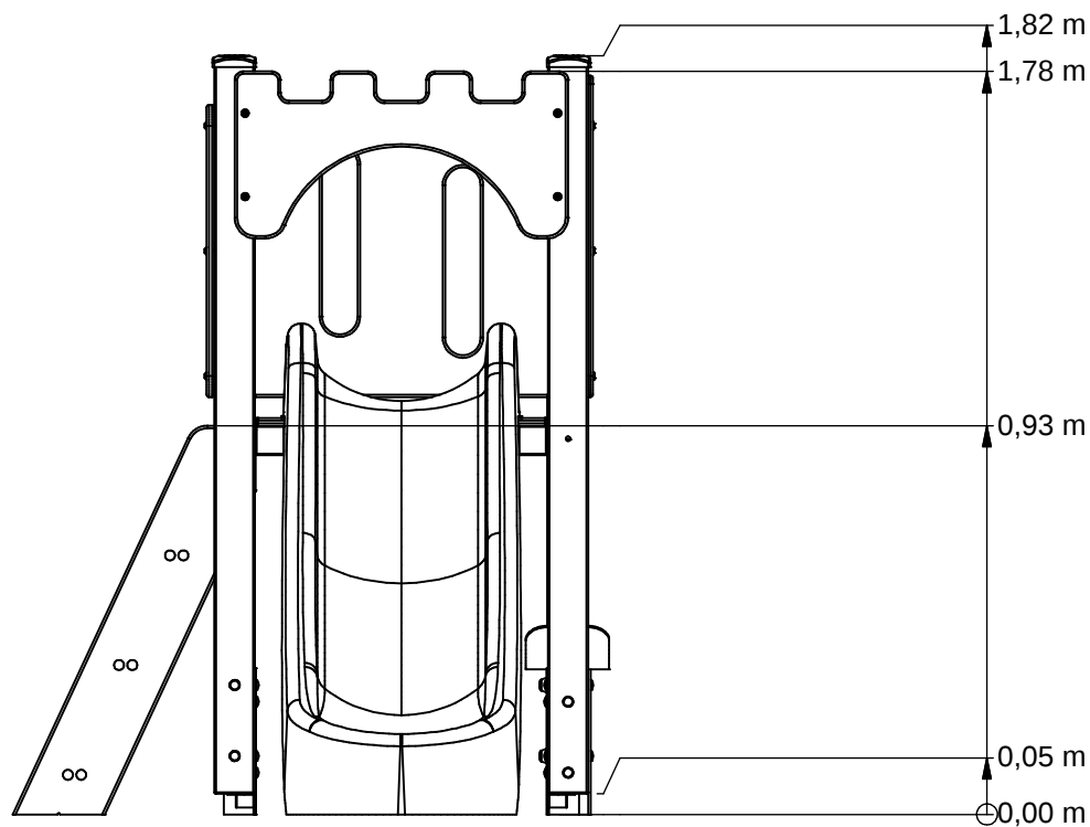
Voor (Front)
