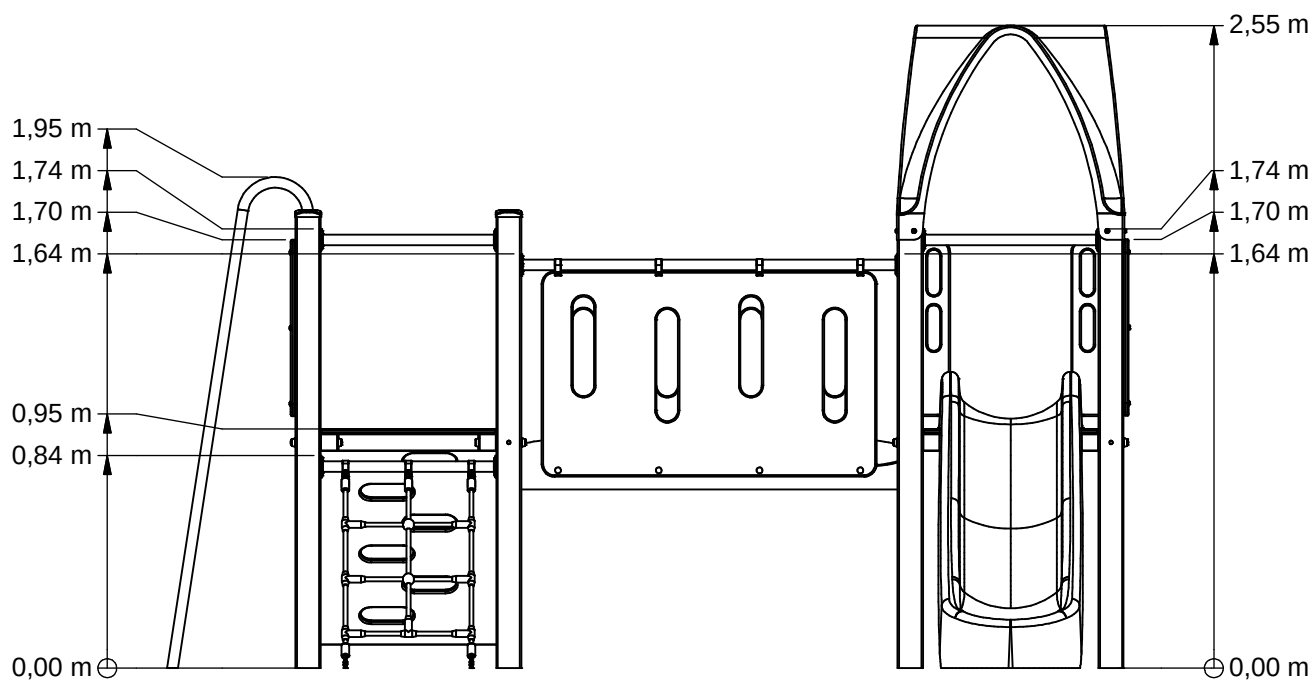
Voor (Front)
