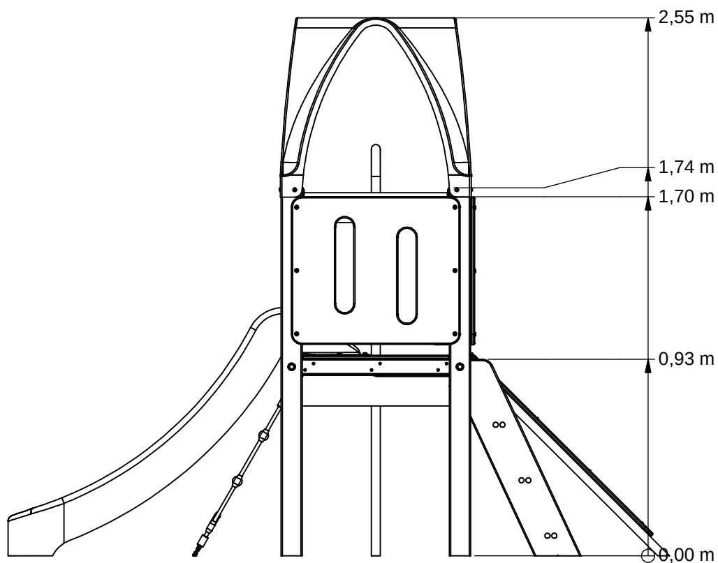
Rechts (Right)
